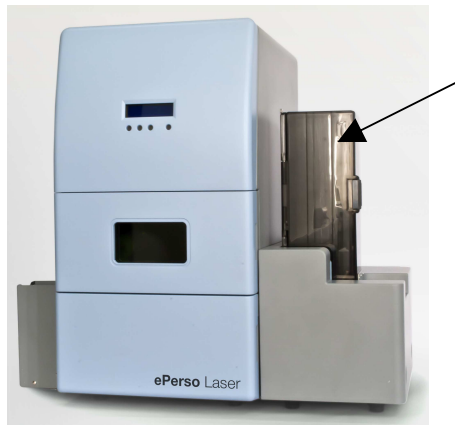
Лоток автоматической подачи с кодировщиками: ISO-7813, ISO-7816, ISO-14443
